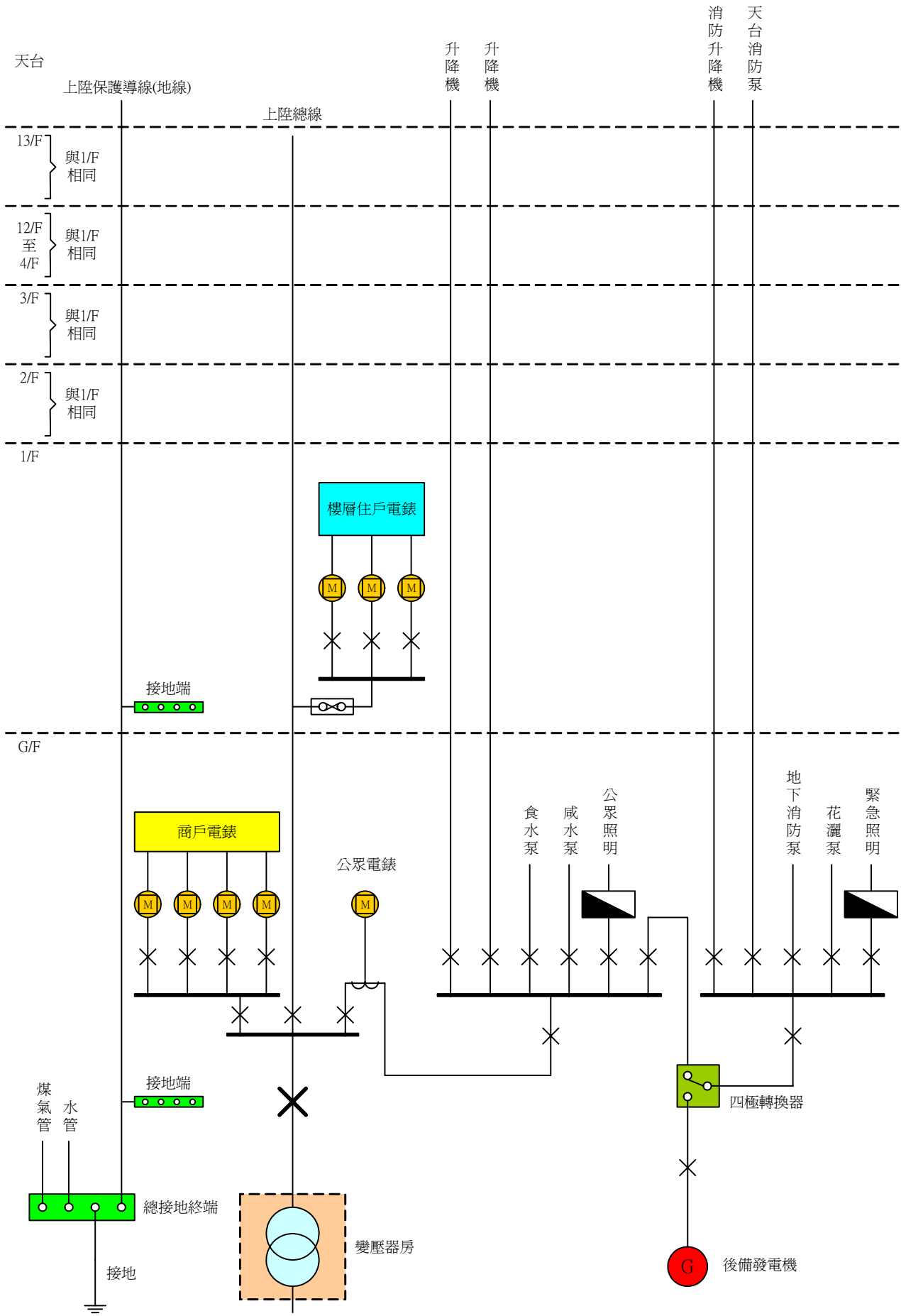
大廈公眾固定電力裝置圖
